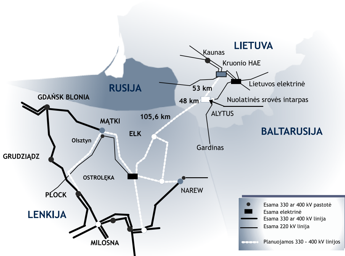
Planuojama elektros energijos perdavimo linija Lietuva - Lenkija
